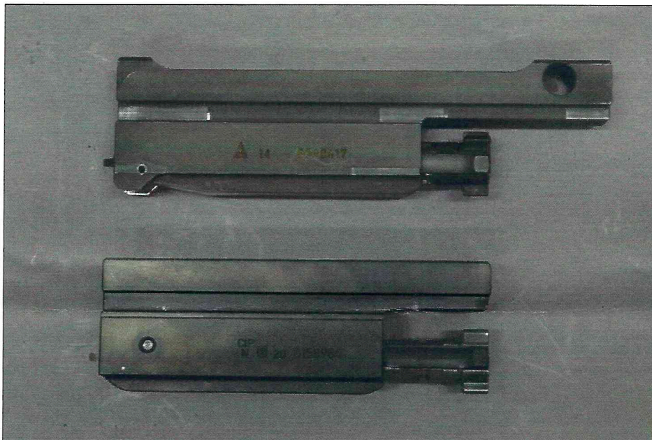
Abbildung 8: Seitenansicht Verschluss mit Steuerkurve, oben der vollautomatische Verschluss „CZ 805 Bren“, unten halbautomatische „CZ Bren 2Ms“
