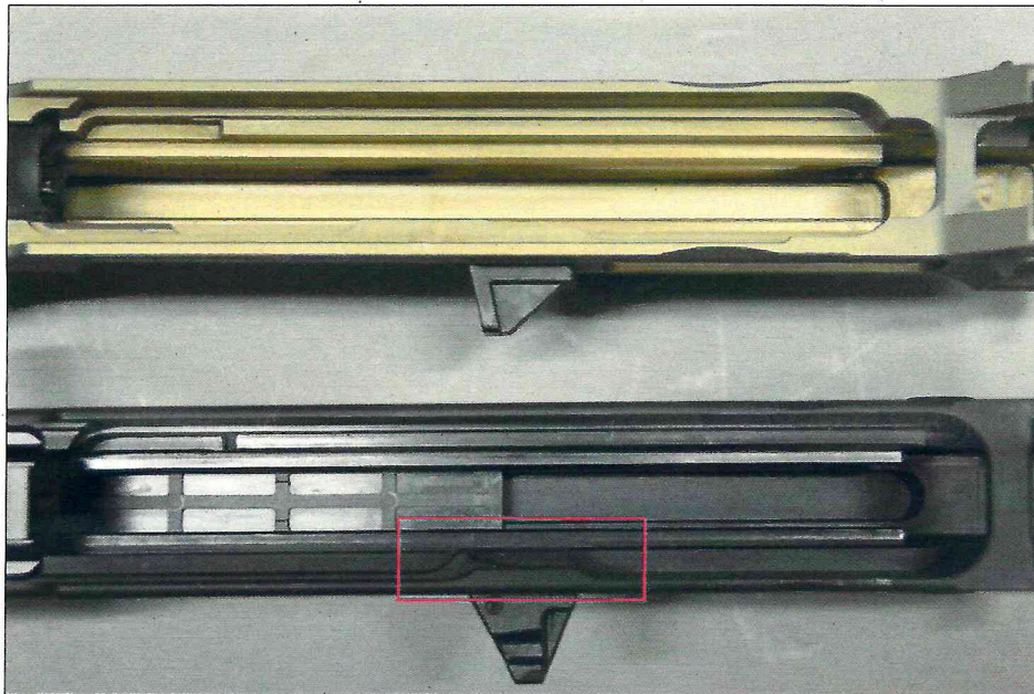
Abbildung 10: Ansicht Gehäuseoberteil-Unterseite mit Öffnung zur Aufnahme des Überstands des Gehäuseunterteil, oben „CZ 805 Bren“, unten „CZ Bren 2Ms“
