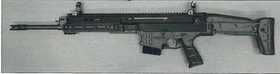
Abbildung 1: „CZ Bren 2Ms“, Ansicht linke Seite
