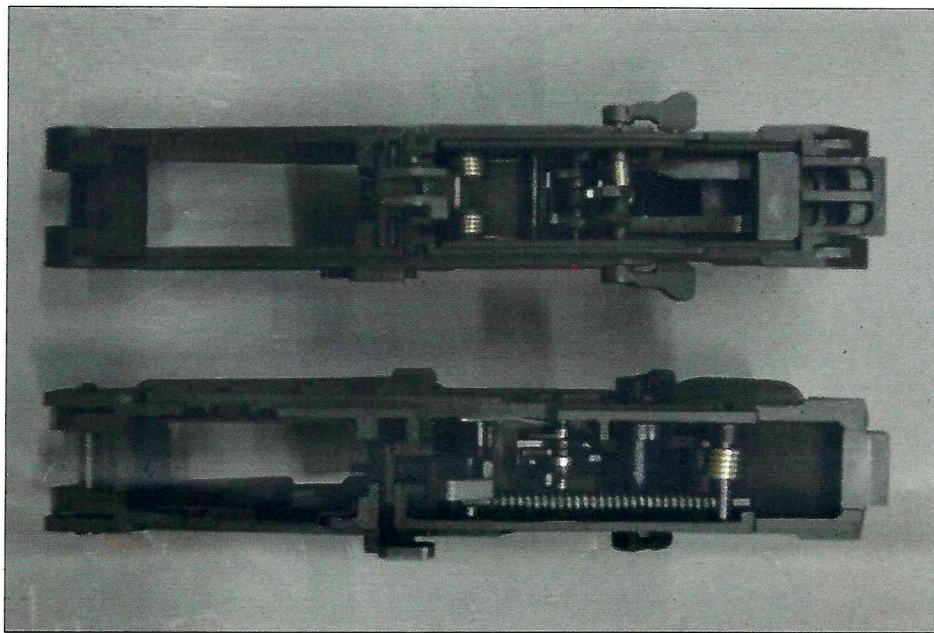
Abbildung 9: Ansicht Gehäuseunterteil mit Abzugsmechanik, oben „CZ 805 Bren“, unten „CZ Bren 2Ms“
