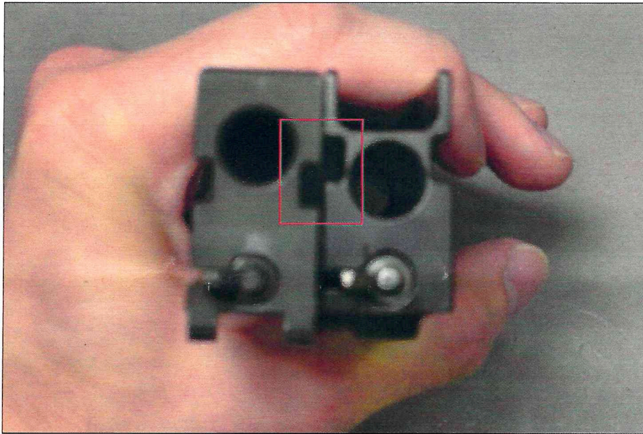
Abbildung 7: Ansicht Verschlussrückseite mit unterschiedlicher Höhe der Ausnehmungen, „CZ Bren 2MS“,
